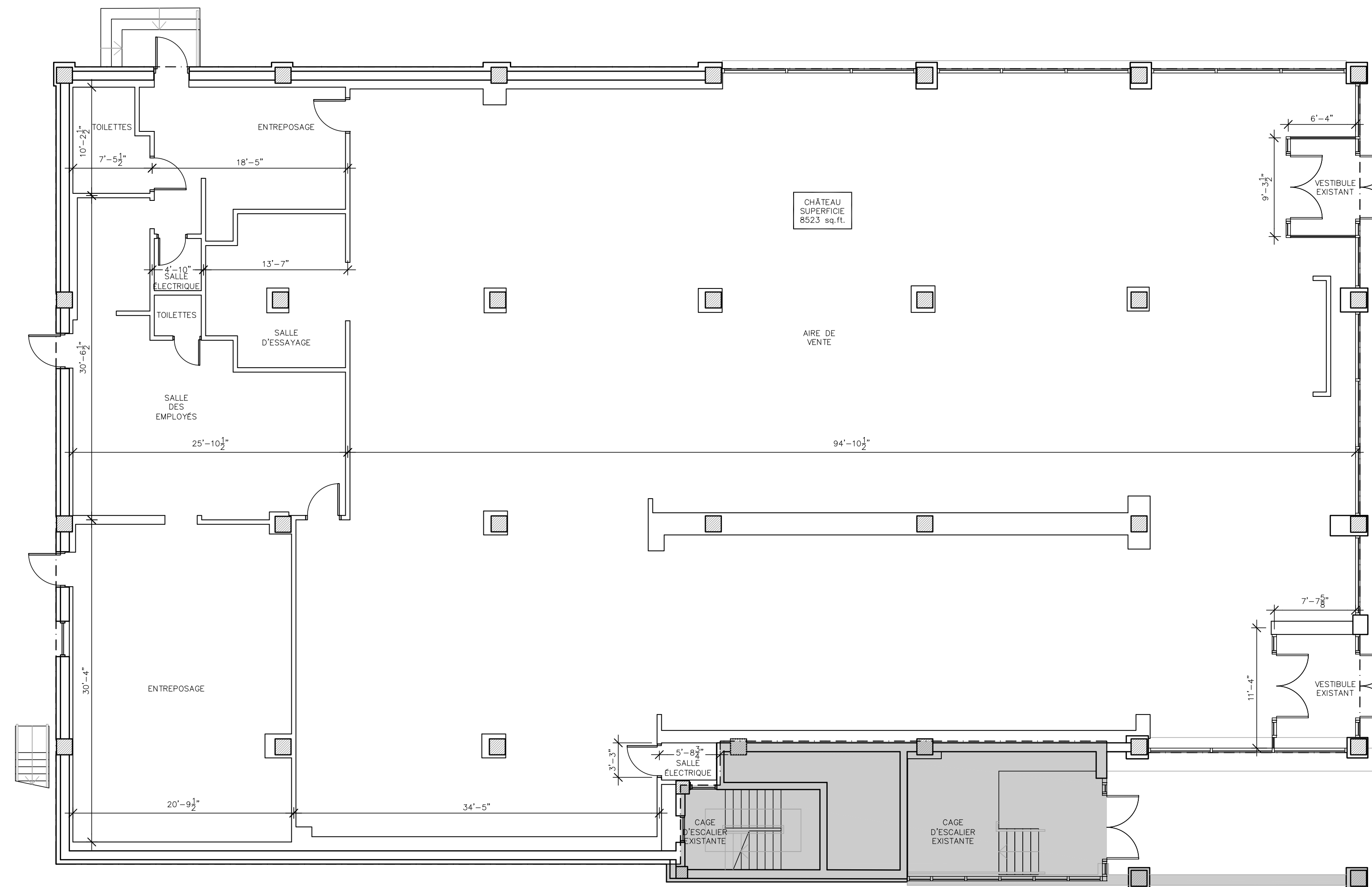
02 PLAN REZ-DE-CHAUSSÉE ÉCHELLE: 1/8"=1'-0"
